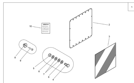
ETB-011022, Tablice ostrzegawcze na rynek francuski od roku prod. 2009!
