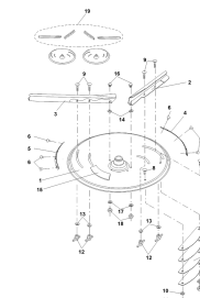
ETB-010987, Tarcza rozsziewająca OSE 27-48
