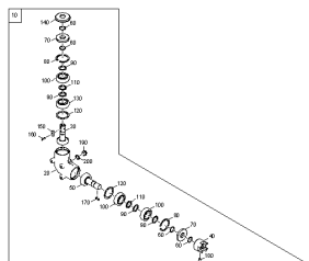
ETB-0000010433, Skrzynia biegów kątowna lewa
