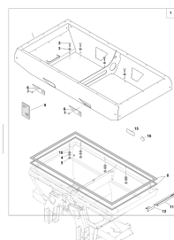
ETB-010980, Nadstawka od roku prod. 2004
