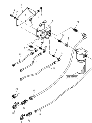
ETB-011005, Blok Comfort do roku prod. 2003
