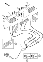
ETB-011021, Oświetlenie od roku prod. 2014
