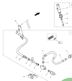
ETB-010993, Hydraulika limiterów Ultra -- od roku prod. 2011
