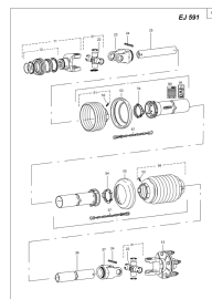
ETB-011026, Wałek przekątnikowy 1 3/8 cala, 6-częściowy, 910 mm EJ591
