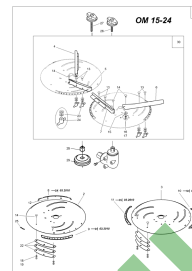
ETB-010990, Tarcza rozsiewająca OM 15-24
