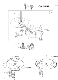
ETB-010988, Tarcza rozsiewająca OM 24-48
