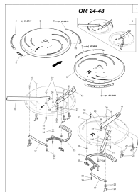
ETB-010989, Tarcza rozsiewająca OM 24-48 (obciążnik wyrównawczy regulowany)
