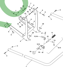
ETB-010994, Rurowy pałak ochronny odchylany
