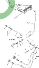
ETB-011004, Siłownik hydrauliczny pojedynczej zasowy
