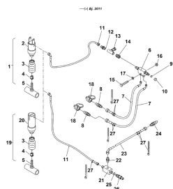
ETB-010992, Hydraulika limiterów Ultra -- do roku prod. 2011
