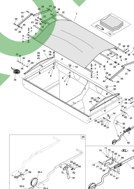
ETB-011015, Składana plandeka
