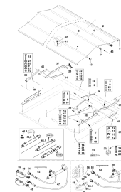
ETB-011016, Składana plandeka hydrauliczna
