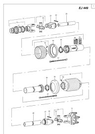
ETB-011025, Wałek przekątnikowy W2102, 760 mm EJ449
