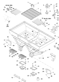
ETB-010977, Rama i elementy montażowe / kratka ochronna
