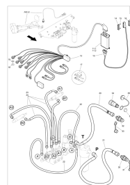
ETB-011012, Pakiet elektroniki Comfort ZA-M Ultra/Profis od 03.2010!
