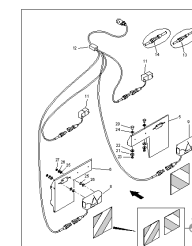
ETB-011020, Oświetlenie od roku prod. 2009 do roku prod. 2013
