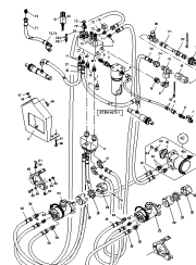
ETB-011008, Hydraulika Ultra Hydro do roku prod. 04.2008
