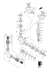
ETB-010998, Przekładnia kąтова
