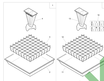
ETB-011023, Ruchome stanowisko pomiarowe
