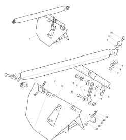
ETB-011029, Ekran rozsiewu krawędziowego lewy
