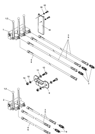
ETB-011010, Zespół dwudrogowy / zespół trójdrogowy
