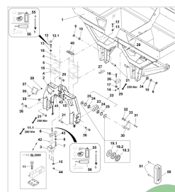
ETB-010981, Rama nakładkowa
