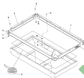
ETB-011014, Nadstawka nad zbiornik S 600
