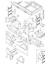
ETB-010979, Blachy ekranujące, trymer, drabina od roku prod. 2004
