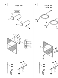
ETB-011019, Oświetlenie przednie do roku prod. 2008!
