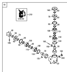
ETB-0000010742, Przekładnia kątowna
