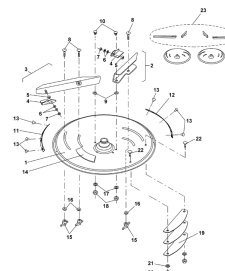
ETB-010986, Tarcza rozsziewająca OSE 18-28
