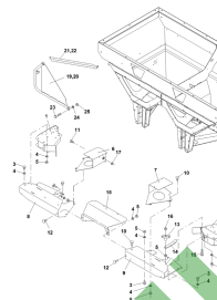
ETB-010978, Blachy ekranujące i trymer do roku prod. 2003
