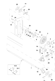
ETB-010999, Wałek mieszadła i jarzmo łańcucha
