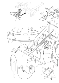
ETB-011028, Ekran rozsiewu krawędziowego obustronny
