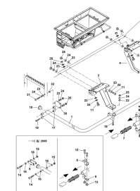
ETB-010995, Rurowy pałak ochronny odchylany, rok prod. 2004
